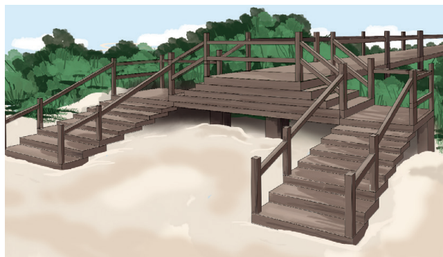
Figura 19. Pasarela en un proyecto de restauración en Telchac-Chixchulub. Se instaló una pasarela en forma de "V" en el frente de playa de los condominios Royal Beach 1, con una elevación aproximada de 50 cm. También se cercó el área revegetada con puntales de madera unidos por cuerda. Fotos: Gabriela Mendoza.
