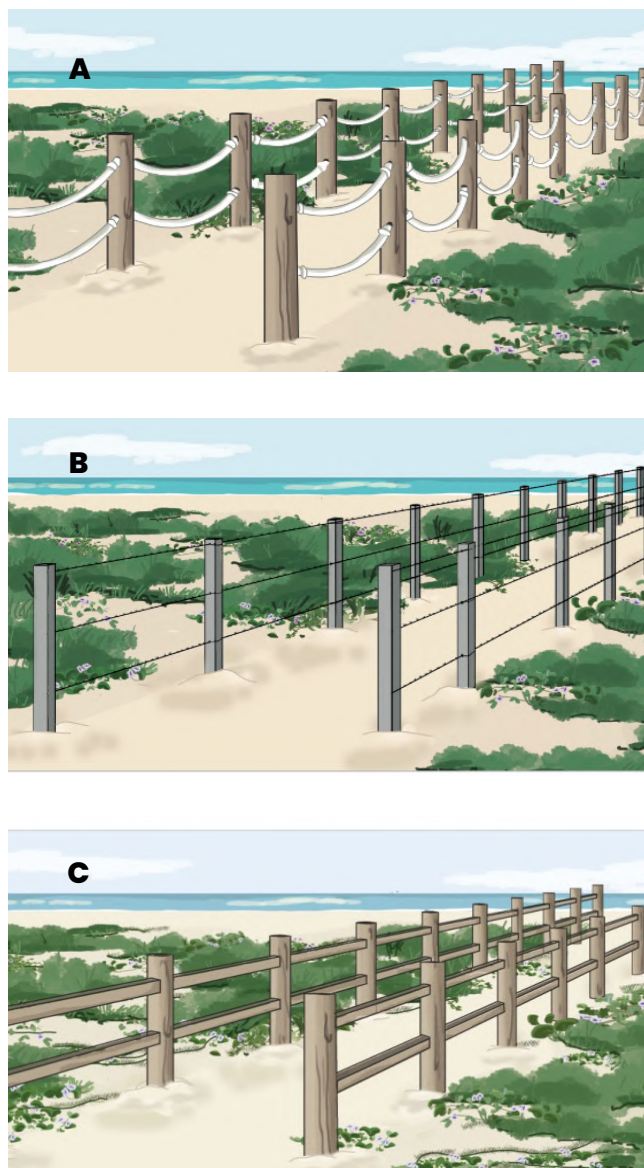
Figura 16. Cercos de protección de la vegetación de dunas costeras. A) Cerco de madera con cuerda; B) Cerco de postes de concreto con alambre de acero inoxidable, C) Cerco de postes y travesaños de madera.
