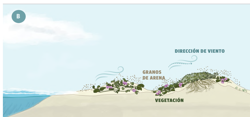
Figura 1. Esquema de la formación de dunas costeras progradante o creciente, en las que la vegetación funciona como obstáculo. A) Interrupción del movimiento de arena por raíces y tallos de plantas; B) Acumulación de arena a causa de las raíces y los tallos enterrados de plantas pioneras; C) Aumento en acumulación de arena formando una elevación; estabilización del sedimento por aumento de cobertura y altura de vegetación; D) Desarrollo de cordones de dunas tierra adentro de manera paralela a la primera acumulación de arena.
