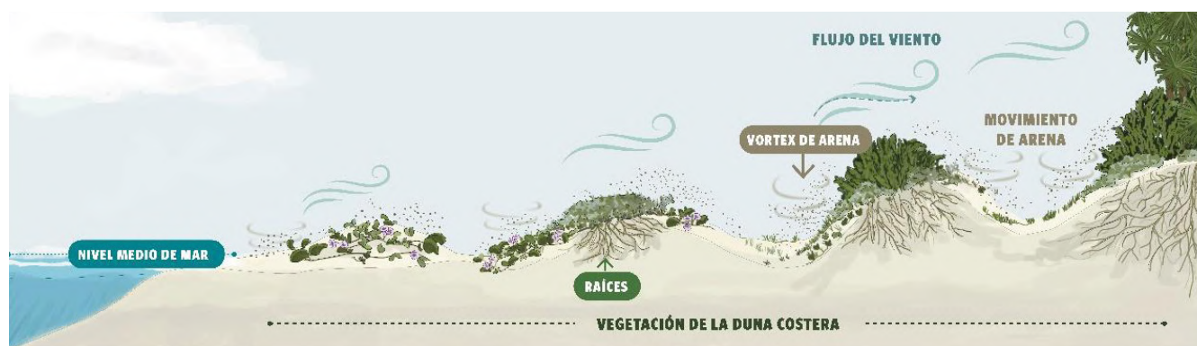
Figura 4. Transporte de granos de arena movidos por el viento proveniente de sotavento. Éstos son obstruidos por las raíces y estructuras de las plantas, lo que genera un vortex de arena (que cambia la dirección del viento), depositándolos y reteniéndolos en dirección barlovento, lo que aumenta la altura y longitud de la duna.
