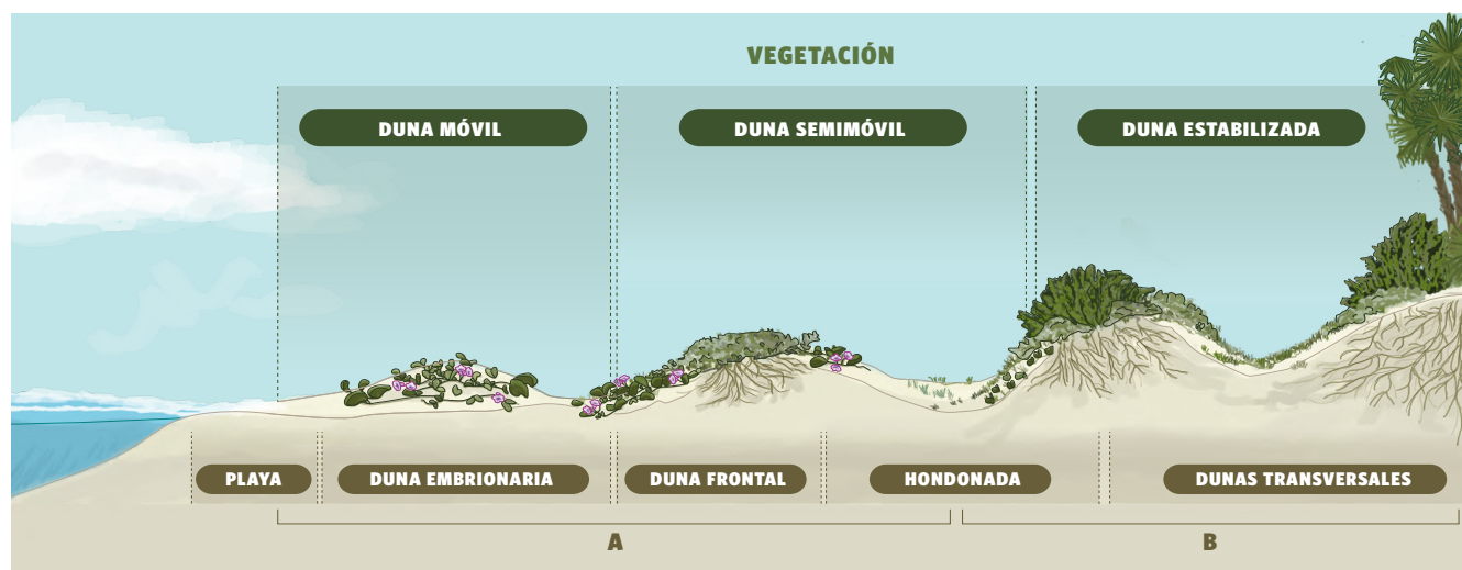
Figura 2. Se observa una zonificación del perfil de dunas, de acuerdo con un criterio topográfico (playa, duna embrionaria, duna frontal, hondonada y dunas transversales) y de vegetación (zona móvil, zona semimóvil, duna estabilizada). A) Indica la vegetación pionera; B) Indica la vegetación de matorral arbustivo.
