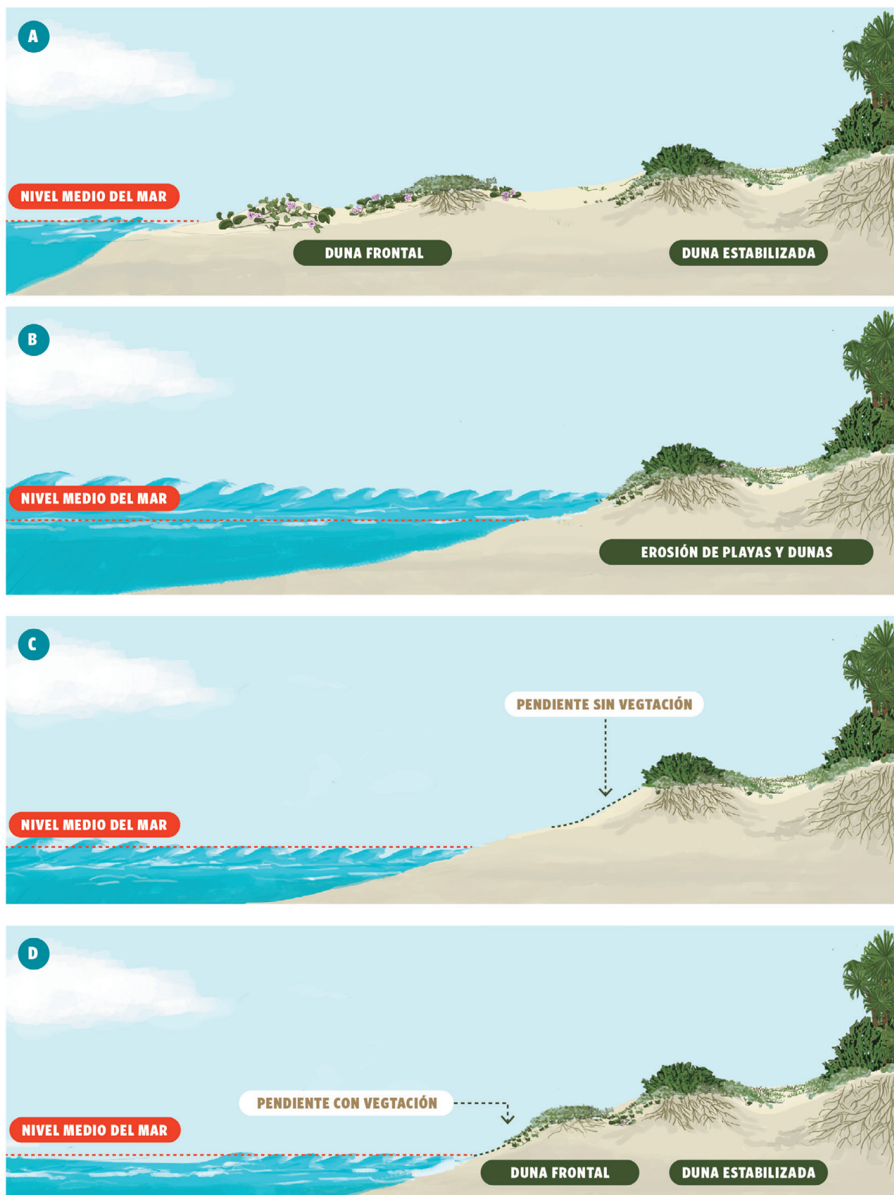
Figura 5. Dinámica y estabilidad de las dunas costeras a lo largo del año. A) Olas moderadas que depositan arena en la playa para formar dunas frontales; B) Aumento del nivel medio del mar durante tormentas que erosionan playas y dunas frontales; C) Temporada de brisas, cuando las olas nuevamente depositan sedimentos en las playas; D) Se generan una vez más espacios ecológicos que permiten el crecimiento de plantas nuevas y la conformación de una duna frontal. Fuente: elaboración propia con base en Hesp (2000).
