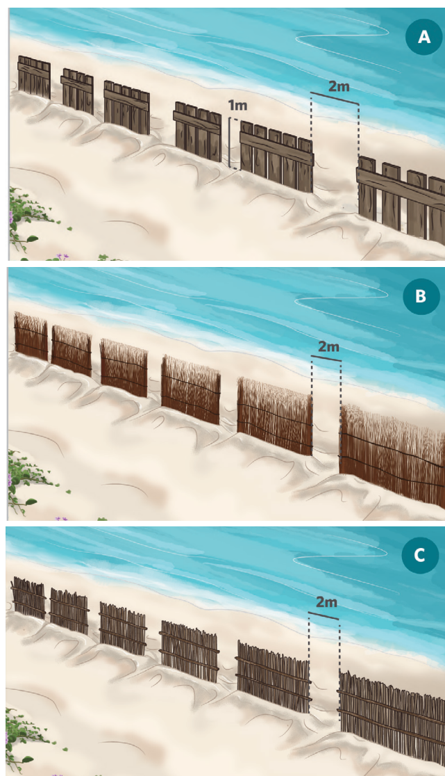
Figura 9. Materiales naturales utilizados para fabricar captadores. A) Captador con tablas de madera; B) Captador con pasto nativo, mimbre o materiales similares; C) Captador elaborado con ramas secas. En todos los casos debe existir un espacio de entre 2 m y 3 m para permitir el paso de tortugas marinas (adultos y crías).
