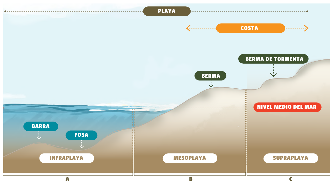
Figura 3. Se observa la zonificación general de playas de acuerdo con el movimiento e intensidad del oleaje y fenómenos naturales. A) Infraplaya (playa sumergida); B) Mesoplaya (zona de rompimiento); C) Supraplaya (zona seca de la playa).
