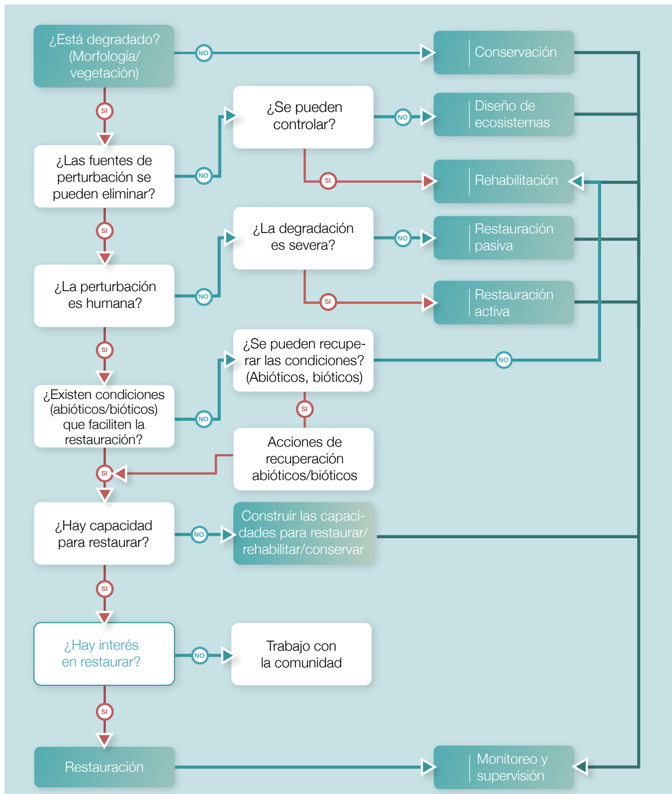
Figura 8. Elementos a tomar en cuenta antes de iniciar un proceso de restauración de dunas costeras. Fuente: elaboración propia con base en Martínez et al. (2016) y Lithgow et al. (2013).
